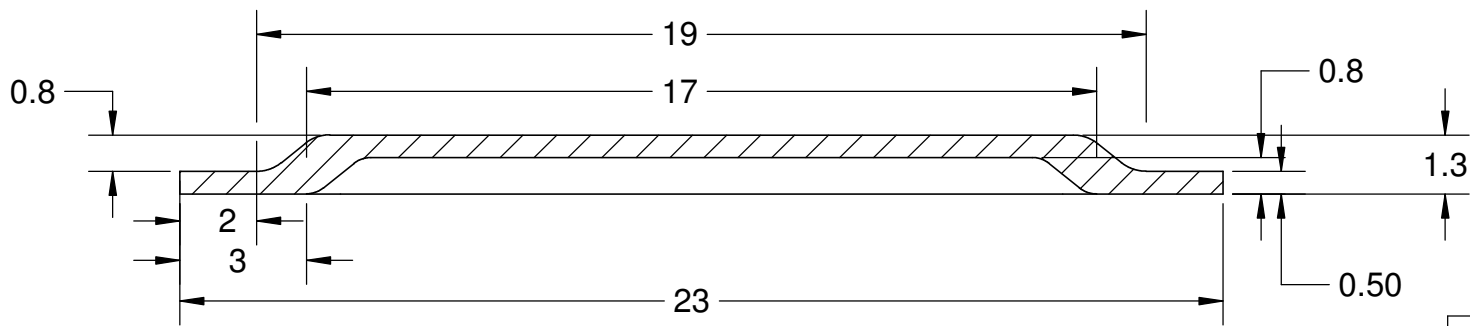
SECTION B-B SCALE 6 : 1
